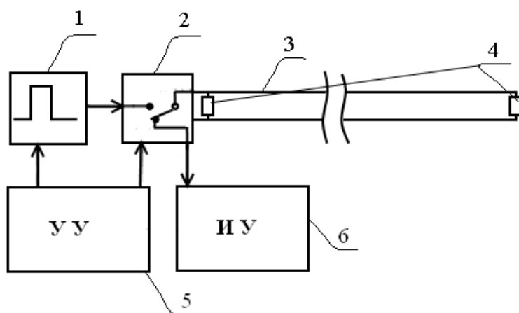
Рис. 1. Схема установки для проведения исследования характеристик чувствительного элемента линейного извещателя пламени: 1 – быстродействующий формирователь импульса; 2 – быстродействующий аналоговый переключатель; 3 – ЧЭ; 4 –согласующее сопротивление; 5 – управляющее устройство; 6 – измерительное устройство
