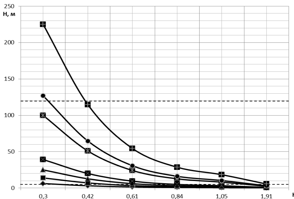
Рис. 1. Зависимость минимального напора на оросителе от коэффициента расхода
