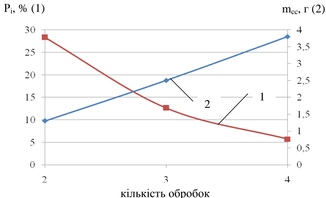
Рис. 1. Втрата маси та витрата сухого складу в залежності від кількості обробок для ясеню обробленої Екосепт: 1 – втрата маси; 2 – витрата сухого складу
