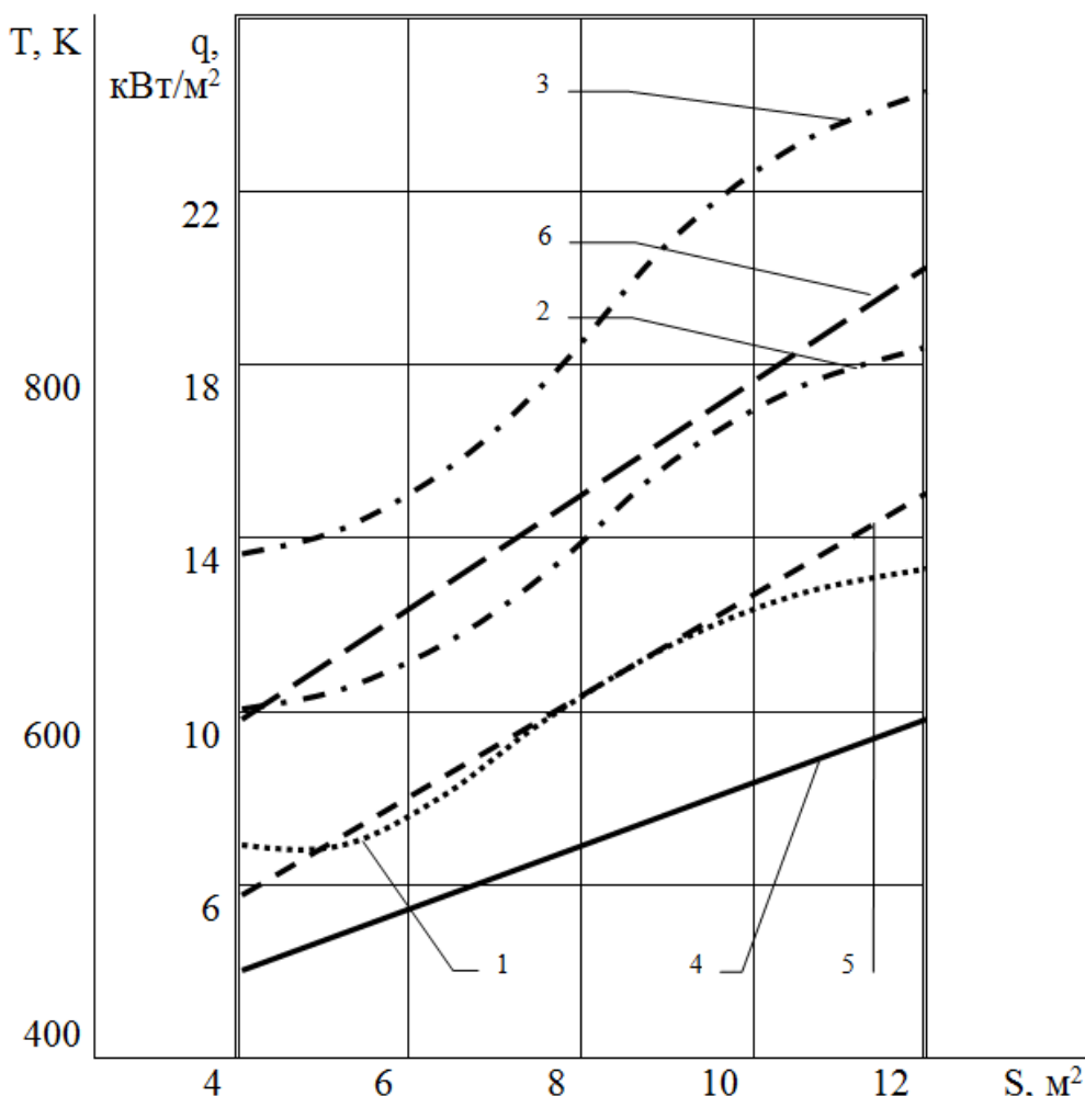
Рис. 2. Залежності променивих потоків (1, 2, 3) і температур (4, 5, 6) від площі перерізу виробітки на стадії повного розвитку пожеж
