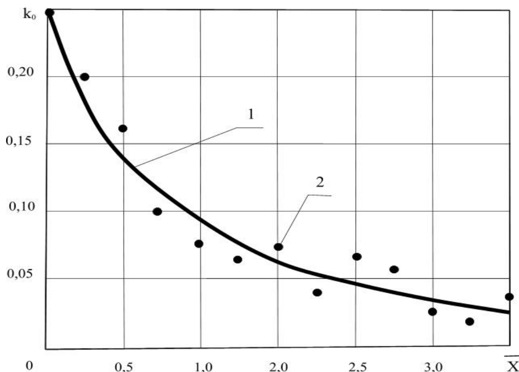
Рис. 3. Залежність коефіцієнта опромінення k_0 від відносної відстані людини у ТЗСО до осередку пожежі \bar{X} : 1 – аналітична; 2 – експериментальна
