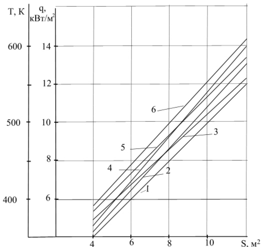
Рис. 1. Залежності променевих потоків (1, 2, 3) і температур (4, 5, 6) від площі перерізу виробітки на початковій стадії розвитку пожежі
