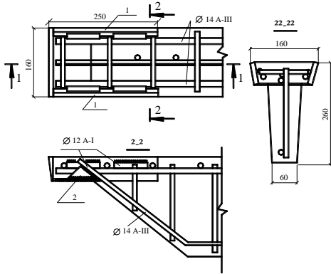
Рис.7. Армування опорного вузла прогону ПЖТ 6-500: 1-сталеві пластина 55x10x250 мм, 2-сталеві пластина 90x5x128 мм
