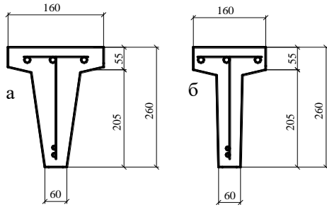
Рис.4. Поперечний переріз прогонів: а-з технологічними ухилами; б-без технологічних ухилів
