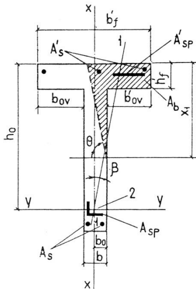
Рис.6. Форма стиснутої зони в поперечному перерізі таврового залізобетонного елемента, що працює на косий вигин: 1-1 — площина дії згинального моменту; 2 – точка докладання рівнодіючої зусиль в розтягнутій арматурі
