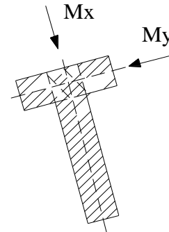
Рис 5. Спрощена схема роботи прогону на косий згин
