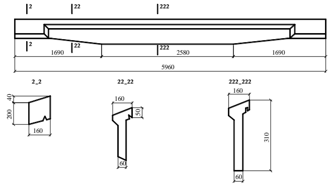
Рис.8. Залізобетонний прогін із скошеною полицею
