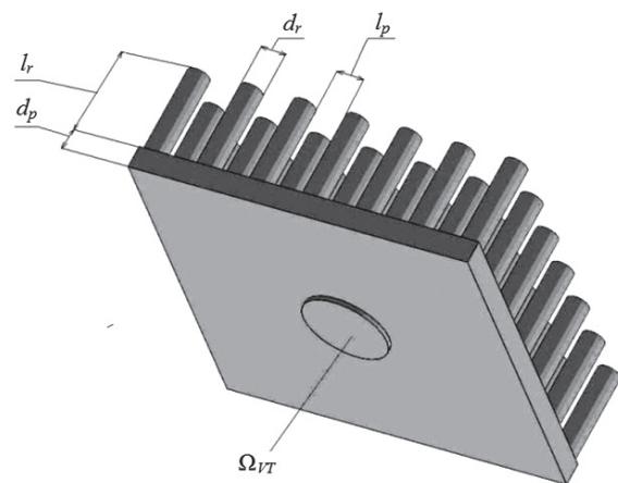
Рис. 1. Тепловая модель штыревого радиатора
