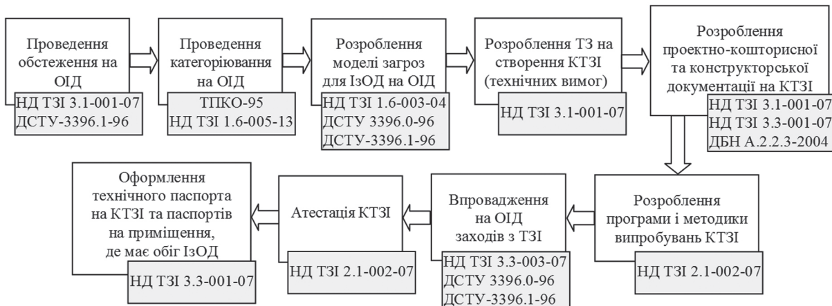
Рис. 4. Порядок виконання робіт створення КТЗІ на ОІД
