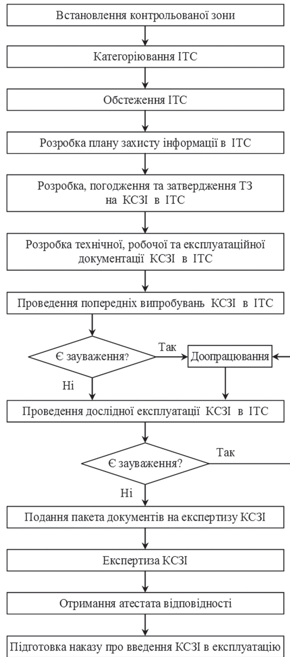
Рис. 3. Порядок створення КСЗІ в ІТС
