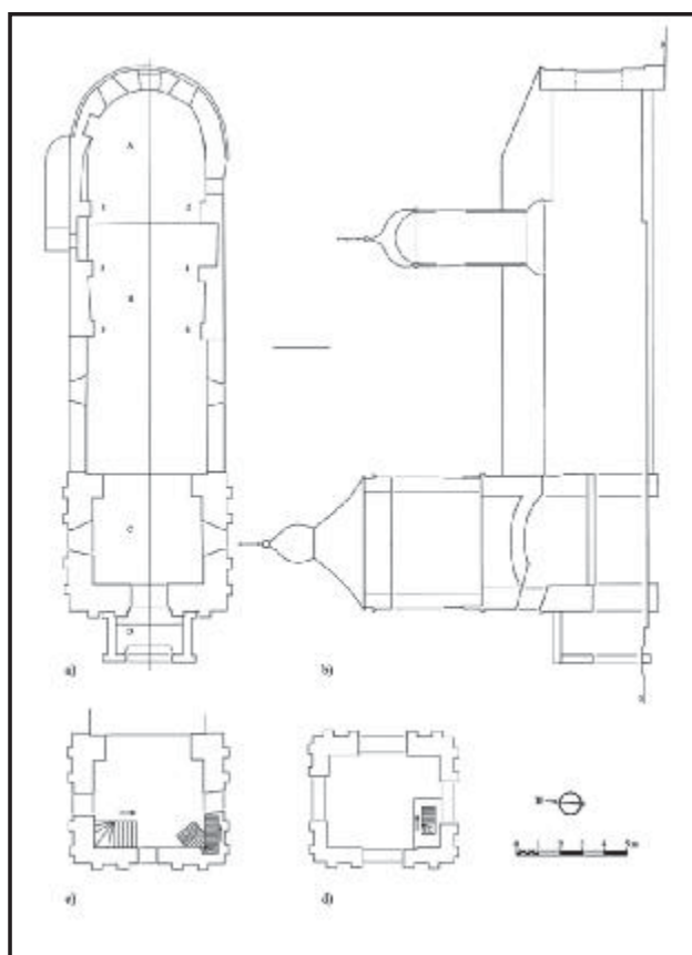
Рис. 1. Грецька церква. План (а) і поздовжній розріз (b). План дзвіниці: II ярус (с), III ярус (d).
