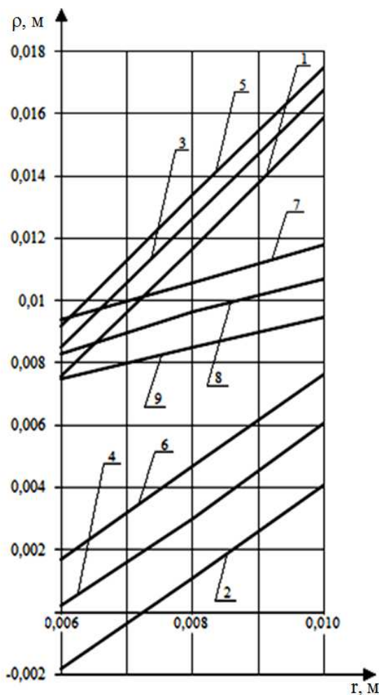
Рис. 2. Залежності переміщення соломини від амплітуди коливань за один оборот ексцентрикового вала, при різних частотах обертання 1, 2 і 7 – графіки залежностей \rho_{\text{вг}} = f(r) , \rho_{\text{вз}} = f(r) і \rho = f(r) при \omega_1 = 45 \text{ c}^{-1} ; 3, 4 і 8 – графіки залежностей \rho_{\text{вг}} = f(r) , \rho_{\text{вз}} = f(r) і \rho = f(r) при \omega_2 = 50 \text{ c}^{-1} ; 5, 6 і 9 – графіки залежностей \rho_{\text{вг}} = f(r) , \rho_{\text{вз}} = f(r) і \rho = f(r) при \omega_3 = 55 \text{ c}^{-1}
