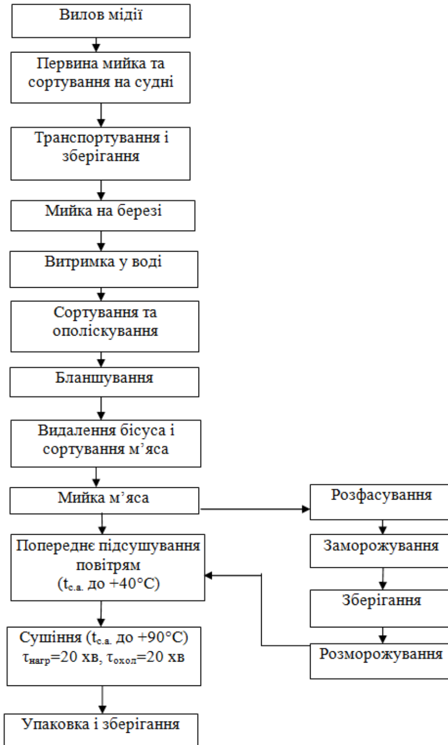
Рис. 1. Технологічна схема виробництва сушеного м'яса мідії.
