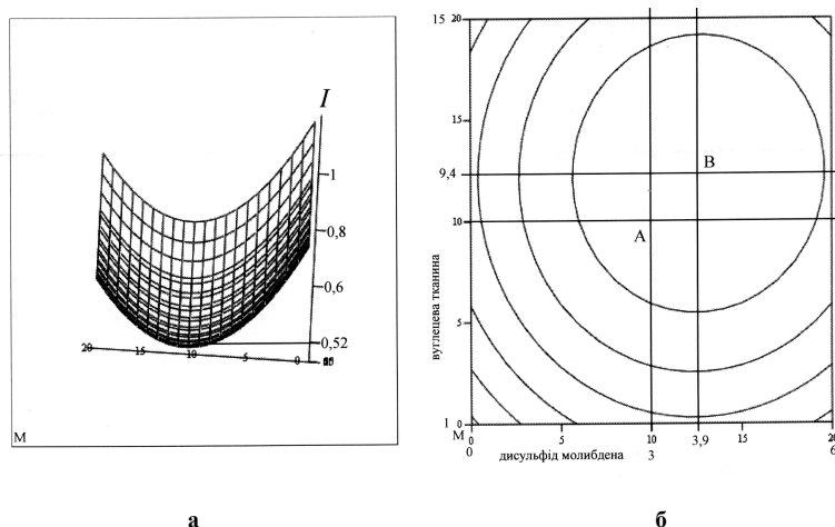
Рис. 4 – Графічна інтерпретація математичної моделі інтенсивності зношування (а) і двовірний переріз функції f(X_i, Y_i, Z_i) при Z_k = 0
