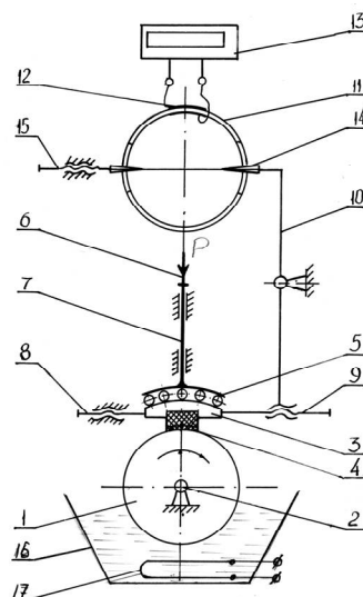
Рис. 3 – Схема приладу для вимірювання моменту тертя:
