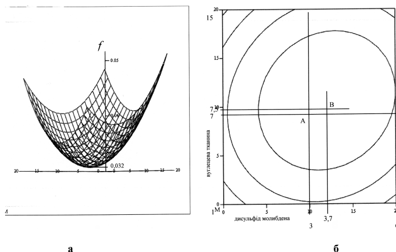
Рис. 5 – Графічна інтерпретація математичної моделі коефіцієнту тертя (а) і двовірний переріз функції f(X_1, Y_1, Z_1) при Z_k = 0
