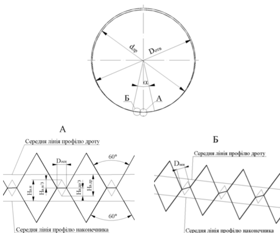
Рис. 4 – Схема утворення контактних площадок між поверхнями струмопідвідного наконечника і зварювального дроту: а – у точці максимального притиску; б – з відхиленням від вертикальних вісей симетрії дроту і наконечника
