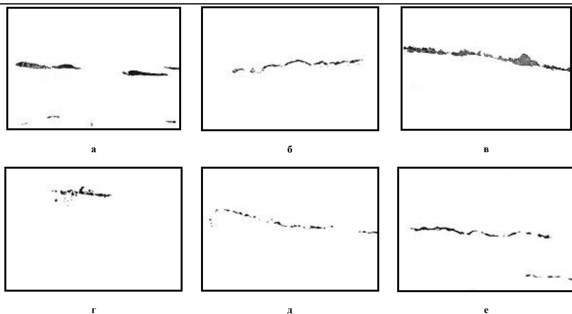
Рис. 2 – Неметаллические включения ( \times 500 ) в холоддеформированной проволоке (суммарное относительное обжатие бунтового проката 85,9 %)
