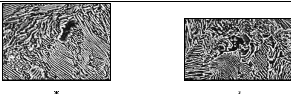
Рис. 3 – Локальная структура бунтового проката из стали S82D вблизи неметаллических включений: а, б – \times 1500 ; в-з – \times 5000 \times 3
