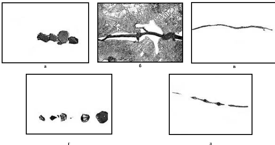
Рис. 1 – Неметаллические включения (× 500) в бунтовом прокате после горячей деформации
