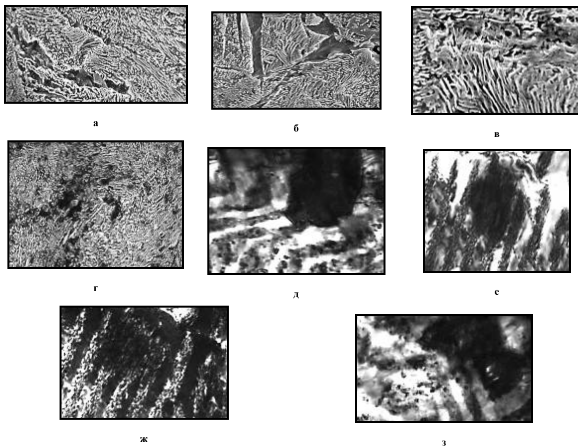
Рис. 4 – Локальная структура стали в холоднодеформированной проволоке вблизи неметаллических включений после различных степеней деформации при волочении: а - г – \times 5000 ; д - з – \times 25000
