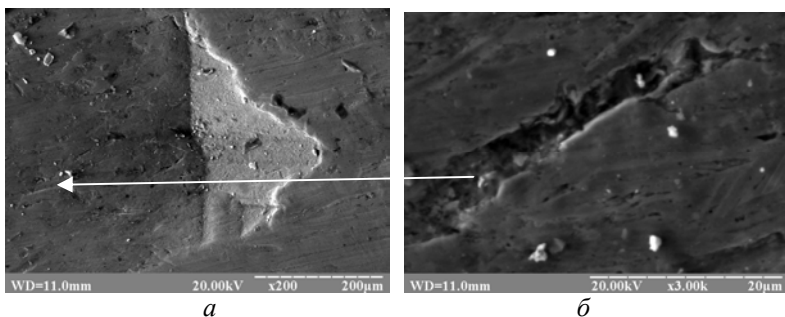
Рис. 2. Мікрофотографії поверхні тертя дискретного покриття 30ХГСА+Л+А після гідроабразивного зношування: а – загальний вигляд дискретної ділянки; б – борозенка на поверхні дискретної ділянки
