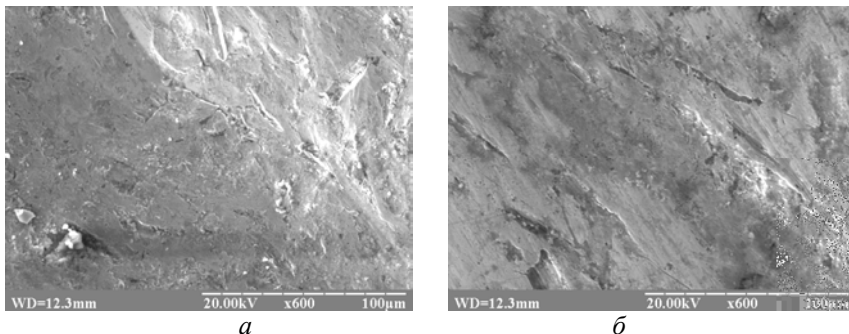
Рис. 4. Мікрофотографія поверхні тертя дискретної поверхні (30ХГСА+Л) після гідроабразивного зношування (зернистість 250-315 мкм): a – внутрішні поверхні лунки; б – поверхня тертя біля лунок
