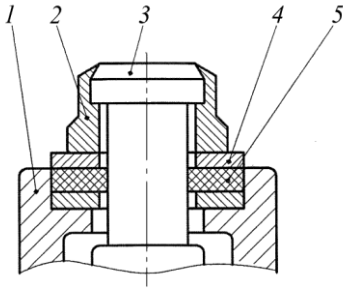
Рис. 12. Демпфирующее устройство в кинематической цепочке подвижной системы ЭМП клапана: 1 – ползун; 2 – стопорная шайба; 3 – шток; 4 – шайба; 5 – пружинный элемент с малой жесткостью
