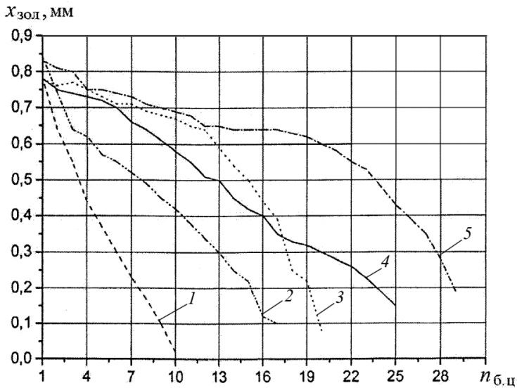
Рис. 8. Зависимость изменения хода золотника в зависимости от количества блок-циклов срабатывания (1 блок-цикл соответствует 20000 циклів) для п'яти клапанів: 1, 2, 3, 4, 5 – номера клапанов
