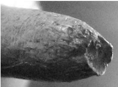
Рис. 10. Усталостные изломы стержневых элементов ЭМК с приводом типа ДТВ: а – материал VT5-1; б – материал АК4-1; в – материал VT1-0
