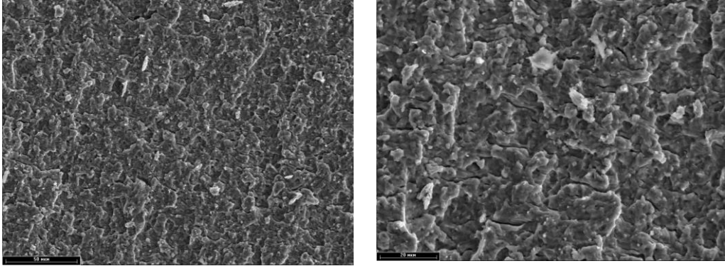
Рис. 11. Фрактограммы усталостных изломов штоков ЭМК из материала ВТ5-1: a – увеличение в 500 раз; б – увеличение в 1000 раз
