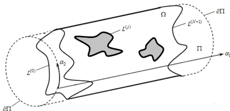
Рис. 1. Циліндрична оболонка з множиною включень довільної конфігурації та зовнішньою границею довільної форми
