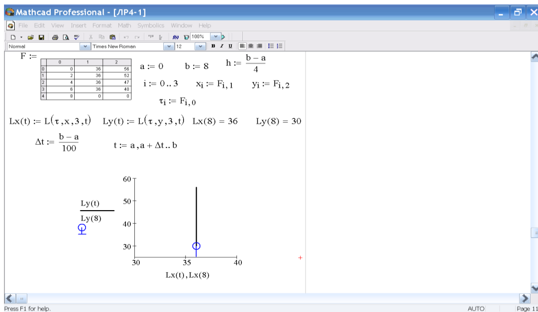
Рис. 1. Комп'ютерна реалізація задачі 1 в MathCAD
