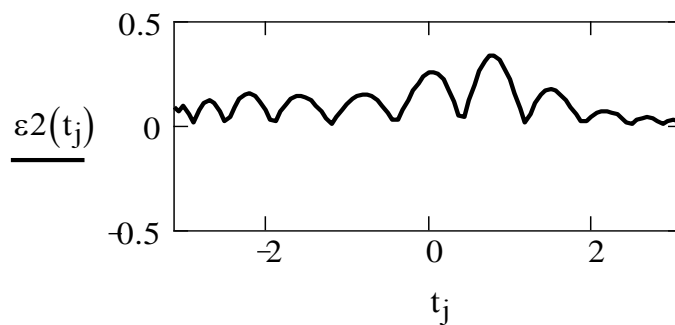
Рис. 4. Оцінка похибки наближення інтерполяційного многочлена для коренів многочлена Чебишева
