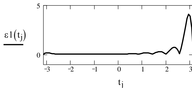
Рис. 3. Оцінка похибки наближення інтерполяційного многочлена для рівновіддалених вузлів
