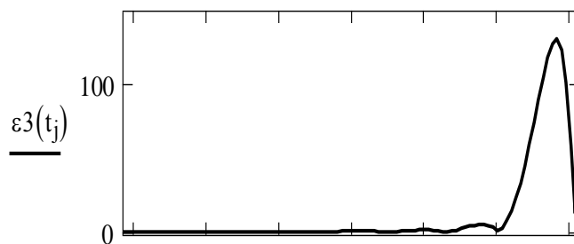
Рис. 4. Оцінка похибки наближення інтерполяційного многочлена для коренів многочлена Чебишева
