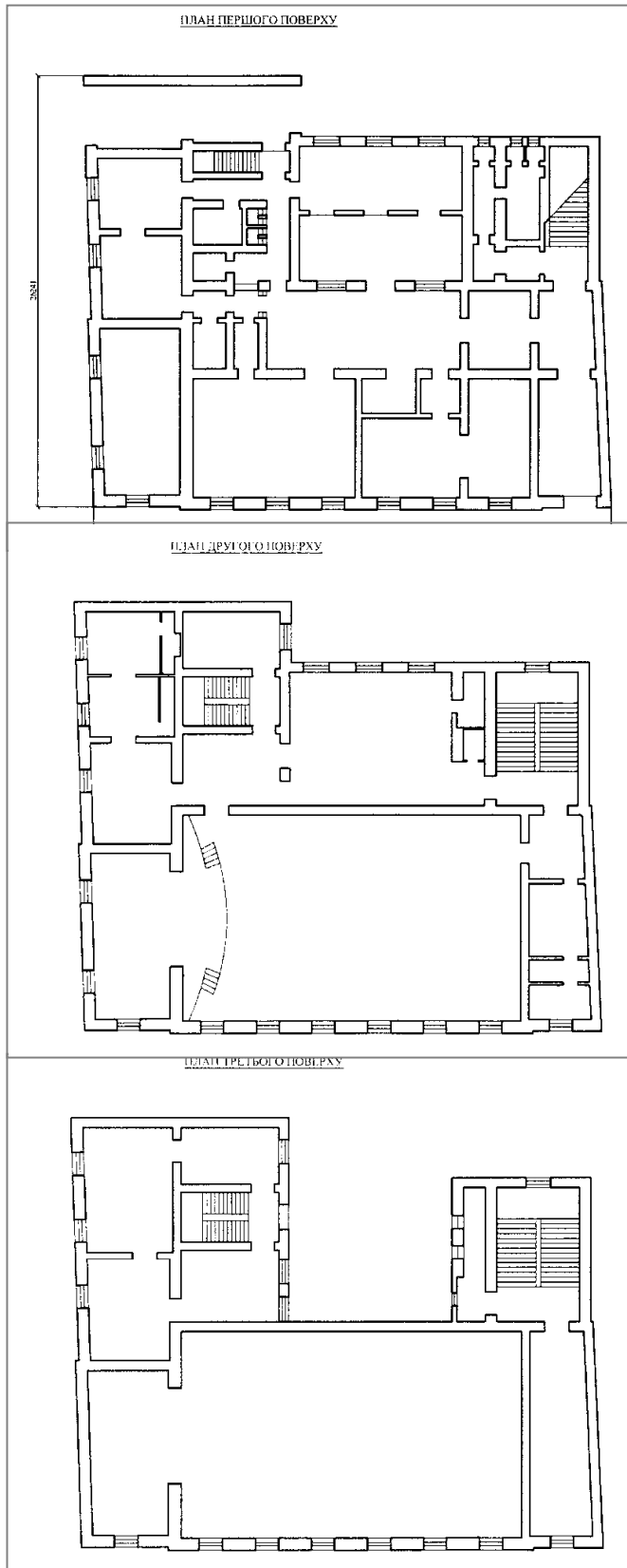
Рисунок 3. Український Народний Дім в м. Стрий. Архітектор І. Левинський. 1897-1901 рр. Обмірні креслення виконані автором у 2007 р.
