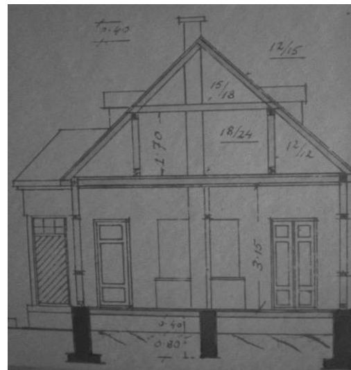
Рис.8. Розріз комбінованого будинку по колишній вул. Бернардинській (Фонд ДАВО)
