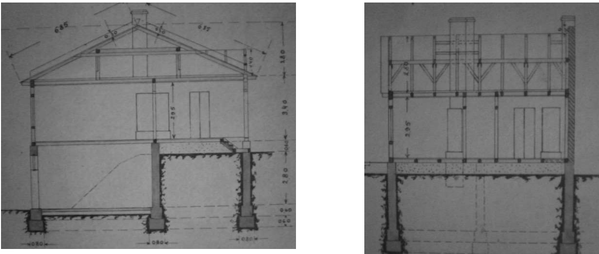
Рис. 5. Поперечний та повздовжній перерізи комбінованого будинку по вул. Гнідавській, 3 (Фонд ДАВО)
