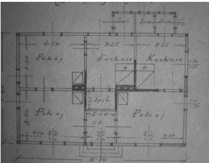
Рис. 7. План комбінованого будинку по колишній вул. Бернардинській (Фонд ДАВО)
