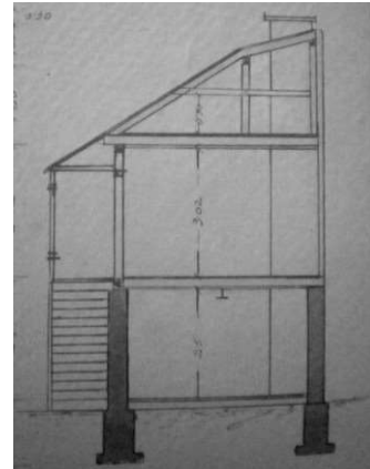
Рис.6. Поперечній та повздовжній перерізи комбінованого будинку по вул. Словацького (Фонд ДАВО)
