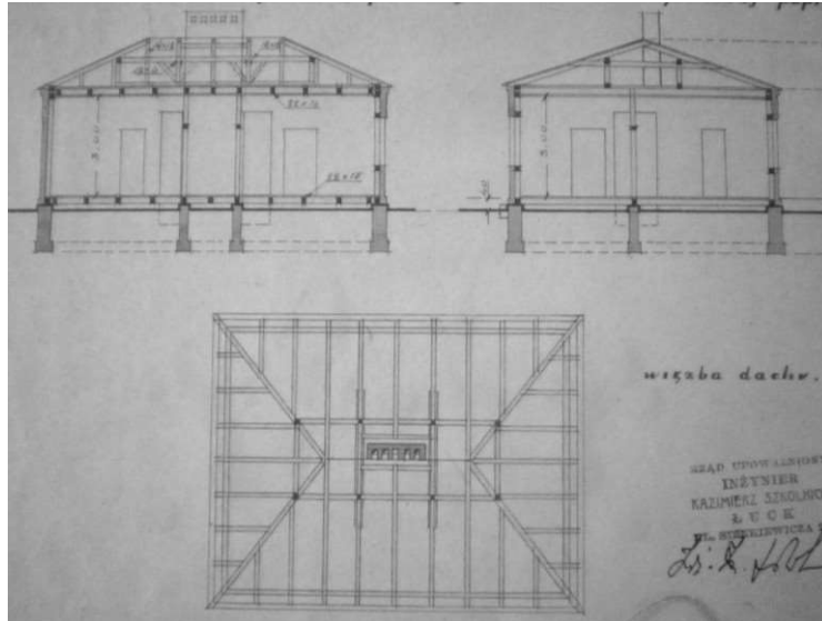
Рис. 11. Повздовжній, поперечний розрізи та план даху будинку по вул. Рівненській (Фонд ДАВО)
