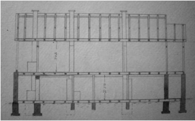
Рис.6. Поперечній та повздовжній перерізи комбінованого будинку по вул. Словацького (Фонд ДАВО)
