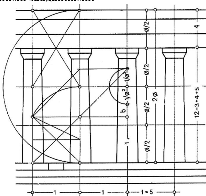
Рис. 1. Геометричні побудови колонади Парфенона [7, с. 45]
