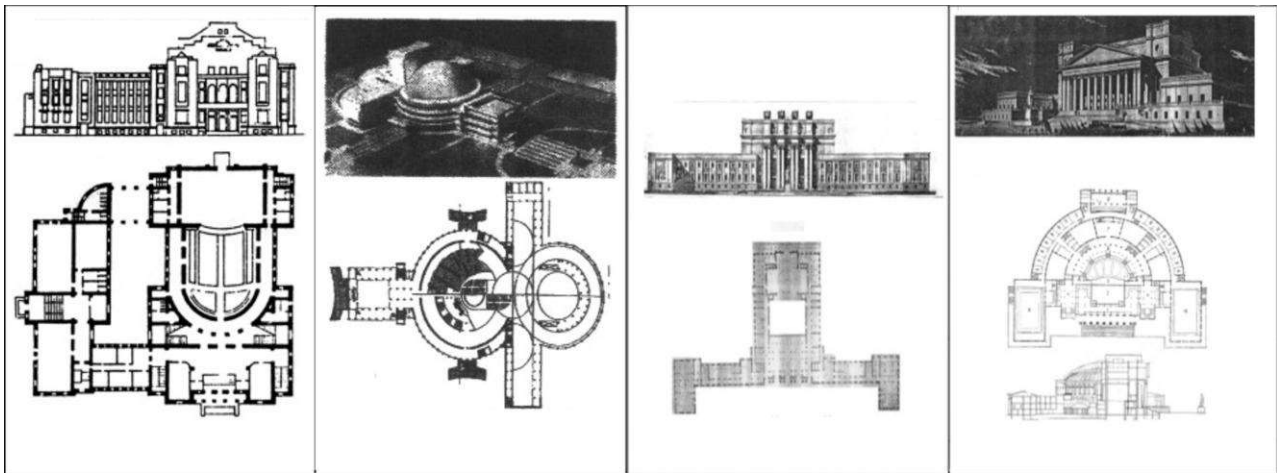
Рис. 1. Дворец культуры по т.п. №1 "Клубстрой" в г. Донецке 1927 г.
