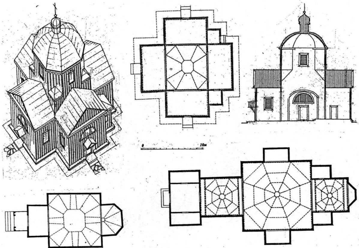
Рис.2. Деякі зразки дерев'яних храмів XIX – п.пол. XX ст.: вгорі - план, розріз та аксонометрія церкви Різдва Богородиці 1835 р. у Лугинах на Житомирищині (реконструкція В.Завади); внизу ліворуч - план Воздзжвиженської церкви 1867р. у Датині Волинської області; внизу праворуч – план Покровської церкви 1928 р. у Бронниках на Рівненщині.
