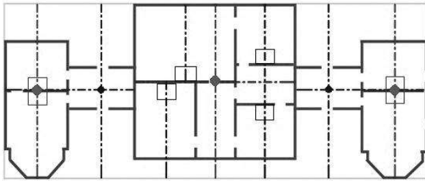
Осевая схема дома Hammond House.
