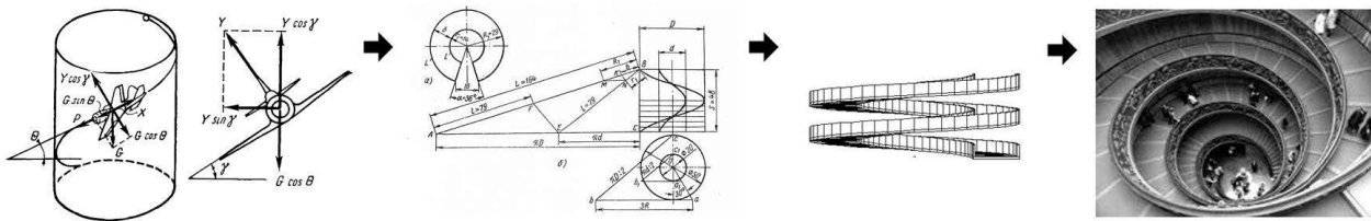
Рис. 3. Концепція формування пішохідного пандуса для огляду експозиції
