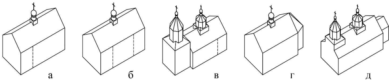
Рис. 3. Група храмів хатнього типу: а) безверхий однозрубний дводільний; б) безверхий однозрубний тридільний; в) одноверхий однозрубний з прибудованою дзвіницею; г) безверхий двозрубний дводільний; д) одноверхий двозрубний з надбудованою дзвіницею. Кресленники автора.
