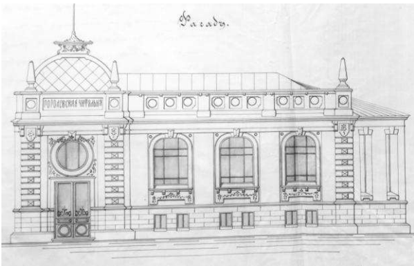
Рис. 3. Проект Гоголівської бібліотеки. 1905р.:
