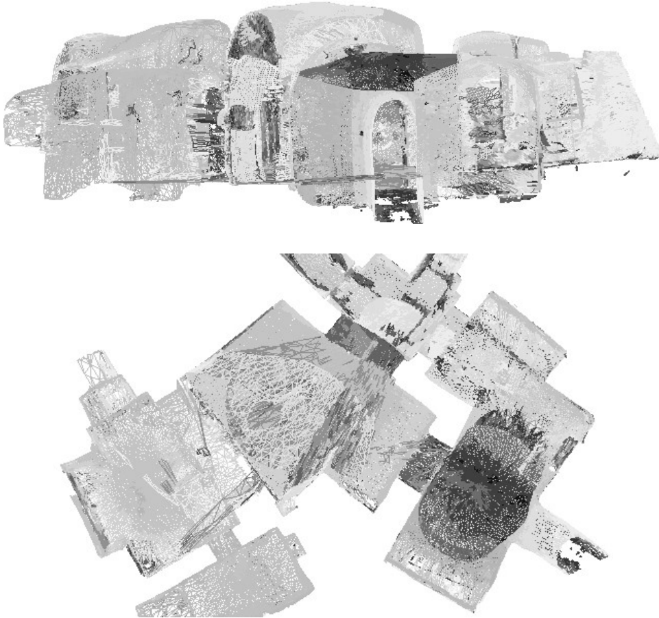
Рис. 3. TIN-модель
