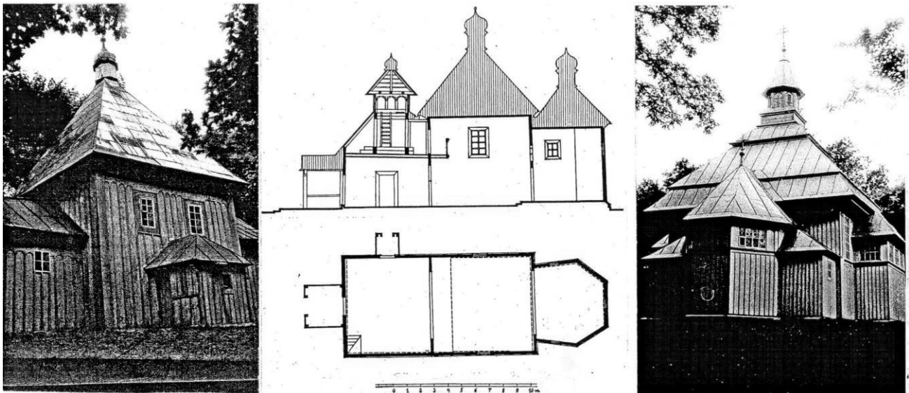
Рис.8. Заміна рубленої конструкції чотирихилого намету каркасною у храмах XVIII-початку XX ст.: ліворуч - у Підлісках Рівненської області, в центрі - у Залізниці Волинської області, праворуч - у Прилуцькому Волинської області.
