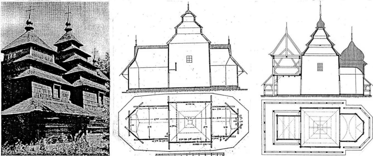
Рис. 3. Збереження чотирикутної в плані форми верхів шляхом влаштування у них додаткових рублених заломів у храмах XVII – XVIII ст.: ліворуч – у Тисовці на Львівщині (за Т. Гевриком); в центрі – у Рогатині на Івано-Франківщині (за М. Драганом); праворуч – у Кутах на Львівщині (за М. Драганом).
