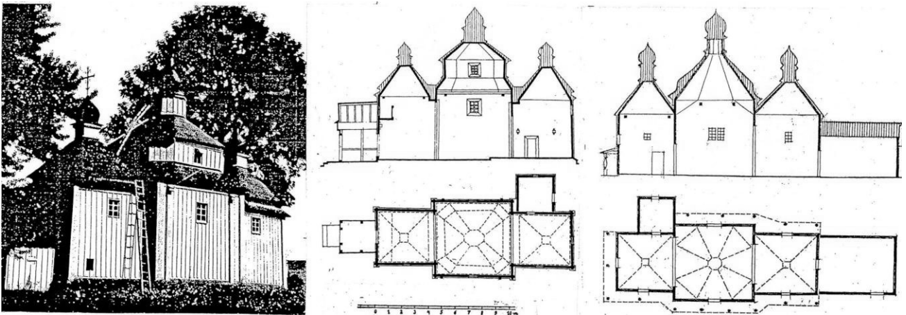
Рис.4. Збереження чотирикутної в плані форми верхів шляхом влаштування їх тільки над меншими за розмірами зрубами бабинця і вітваря у храмах XVII – XVIII ст.: ліворуч і в центрі – у Жубровичах Житомирської області; праворуч – у Старих Хуторах на Вінниччині (за П.Юрченком).
