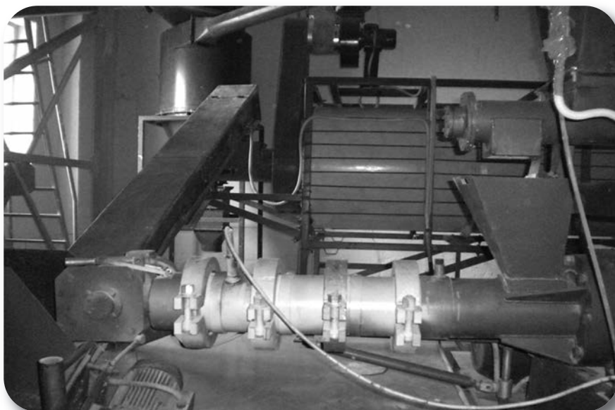
Установка для экструдирования сырья "BRONTO" E-1000
