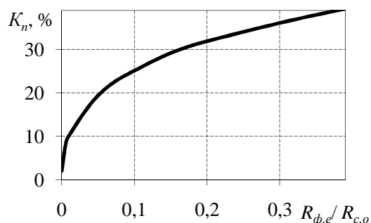
Рисунок 4 – Залежність коефіцієнта проникнення тест-аерозолію крізь респіратор від відношення величин опору фільтрувального елемента і смуги обтюрації
