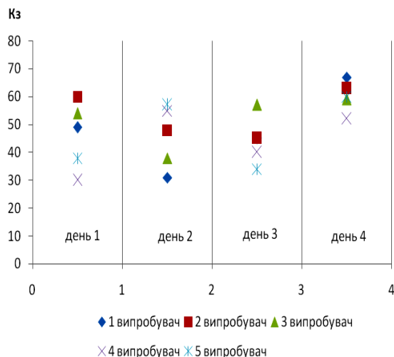
Рисунок 6 – Значення коефіцієнту захисту респіраторів РПА при температурі навколишнього середовища 28 °С
