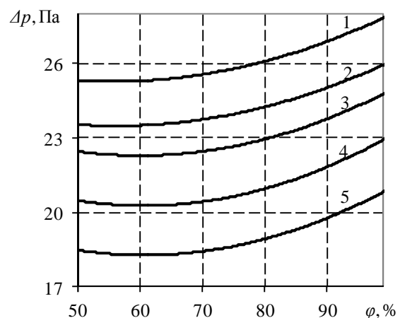
Рисунок 5 – Криві залежності перепаду тиску респіратора типу Лепесток від вологості повітря, при різній температурі навколишнього середовища, °C: 1 – 30; 2 – 26; 3 – 24; 4 – 20; 5 – 16
