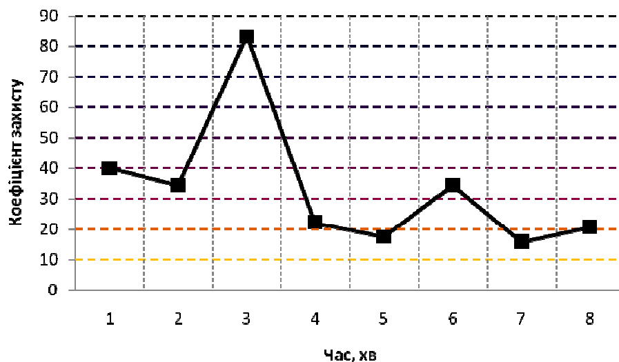
Рисунок 1 – Зміна коефіцієнта захисту респіатора з часом
