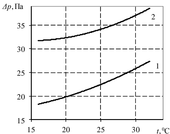
Рисунок 4 – Криві залежності перепаду тиску на фільтрувальному матеріалі від температури:
