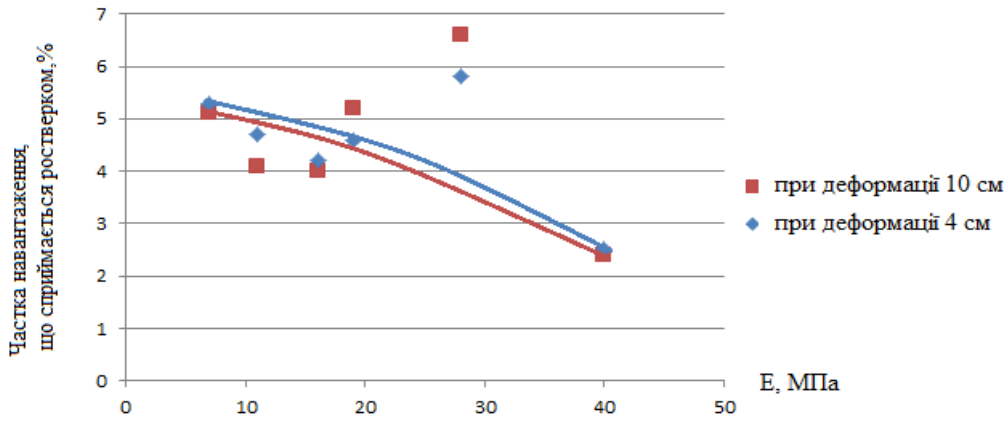
Рис. 3. Залежність частки навантаження, що сприймається ростверком, від модуля деформації
