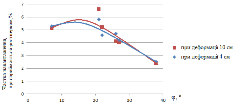
Рис. 2. Залежність частки навантаження, що сприймається ростверком від кута внутрішнього тертя
