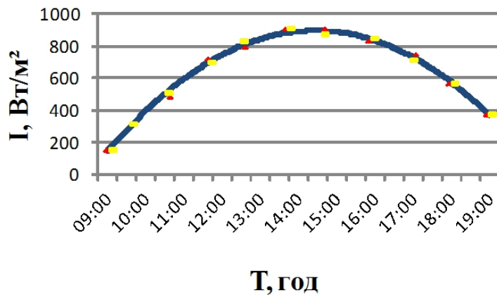
Рисунок 5 – Зміна інтенсивності сонячної енергії I на площину геліоустановки впродовж дня
