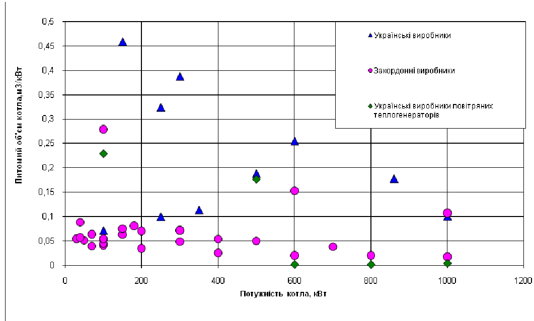
Рисунок 3 – Залежність питомого об'єму водогрійних котлів та повітряних теплогенераторів V/Q , \text{кВт}/\text{м}^3 залежно від їх потужності Q
