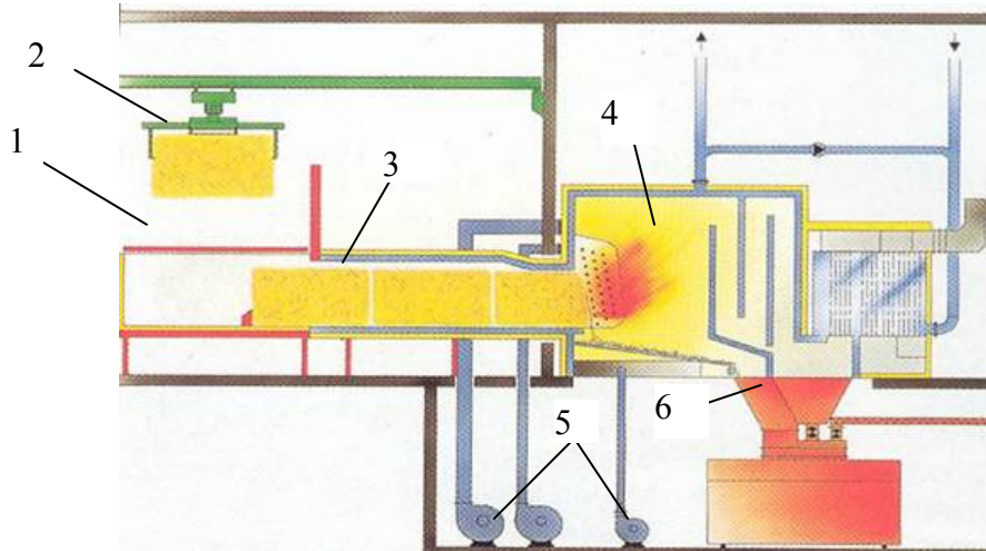
Рисунок 1 – Котел Lin-ka (2, 4, 10 МВт) для "цигаркового" спалювання тюків соломи [10] 1 – склад для зберігання соломи; 2 – під'ємний кран; 3 – система подачі сировини; 4 – котел; 5 – система вентиляторів; 6 – система видалення золи і шлаку
