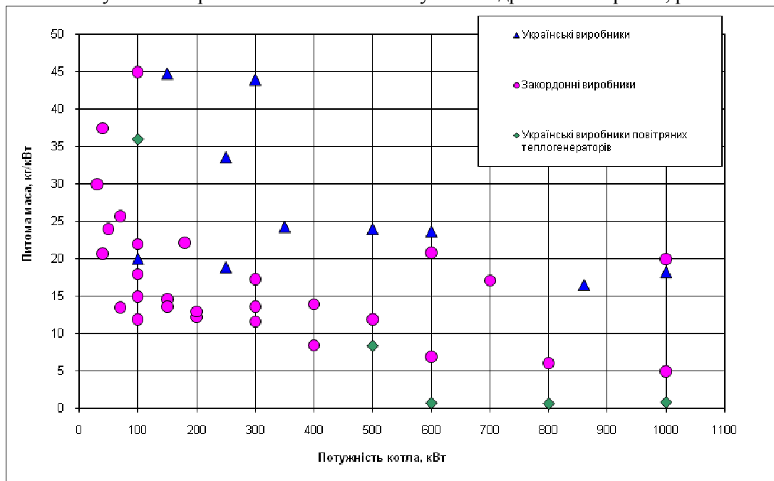
Рисунок 2 – Залежність питомої маси водогрійних котлів та повітряних теплогенераторів M/Q залежно від їх потужності Q
