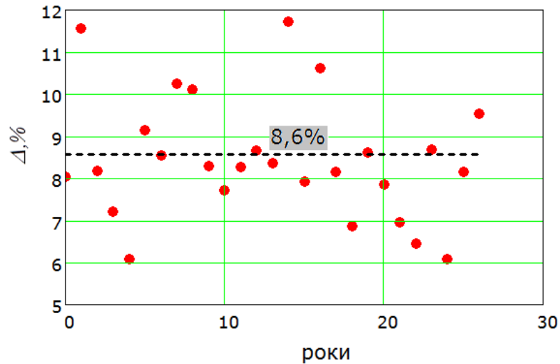
Рисунок 4 – Відхилення з визначення витрати енергії на нагрівання інфільтраційного повітря за опалювальний впродовж 27 років, обчислені з урахуванням та без урахування мінливості метеорологічних факторів
