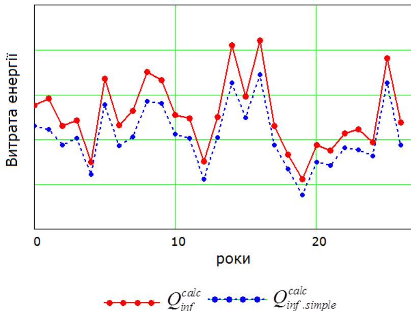
Рисунок 5 – Графіки зміни витрати енергії на нагрівання інфільтраційного повітря за опалювальний період впродовж 27 років обчислені з урахуванням та без урахування змінності метеорологічних факторів
