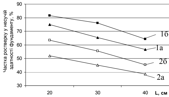
Рисунок 7 – Графік залежності частки, яку складає несуча здатність ростверку у складі підсиленого фундаменту, від довжини паль [1]: 1a і 1б – модель №1 при кроці паль 3d і 6d відповідно; 2a і 2б – модель №2 при кроці паль 3d і 6d відповідно
