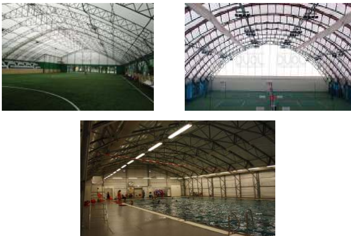
Рис. 1. Швидкозведені каркасні покриття для фізкультурно-спортивних комплексів: а) футбольного поля; б) тенісного корту; в) плавального басейну
