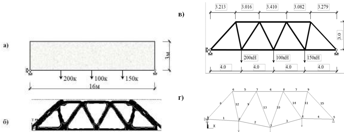
Рисунок 2 – Топологічна оптимізація ферми
