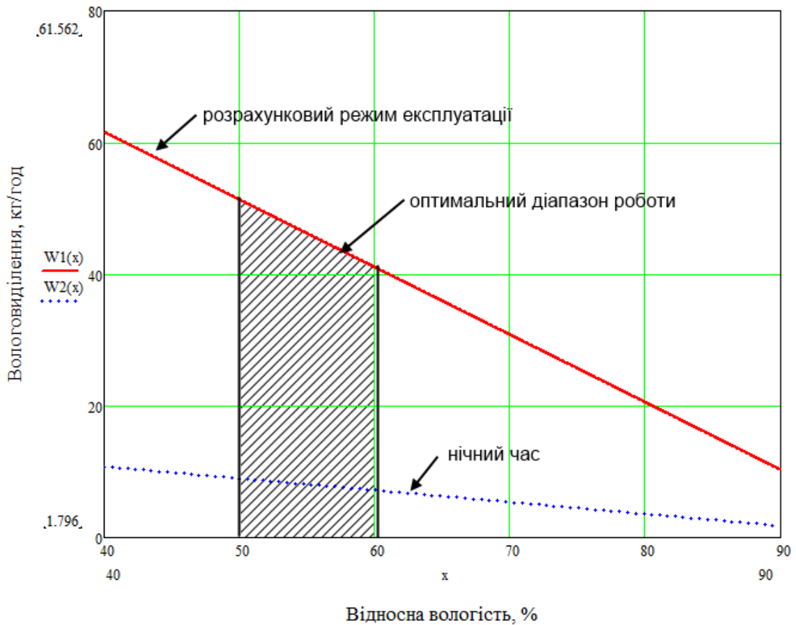
Рисунок 1 – Залежність вологовиділень W , кг/год від відносної вологості x внутрішнього повітря для площі дзеркала громадського басейну 100 \text{ м}^2 (розраховано згідно методики [3])
