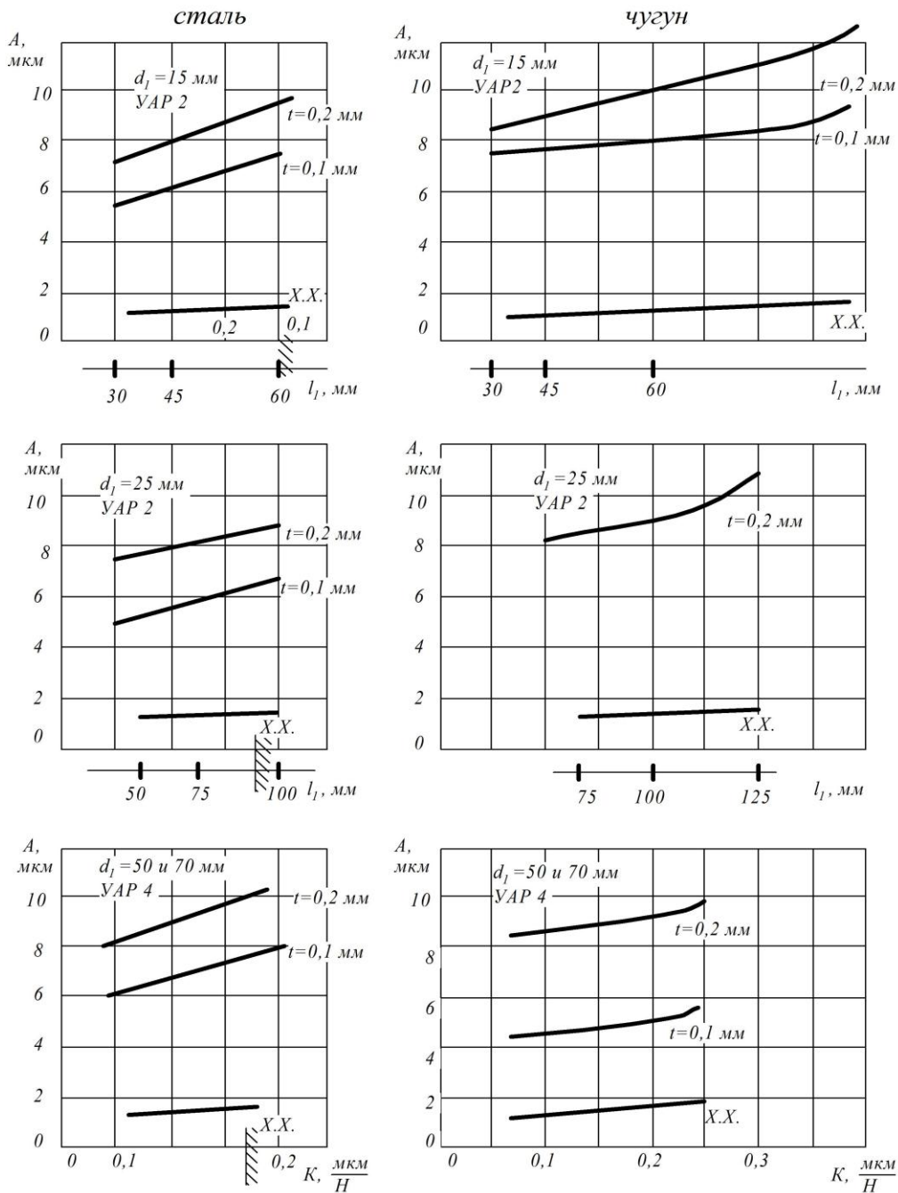
Рисунок 4 – Колебания длинных борштанг при растачивании; X.X. – холостой ход
