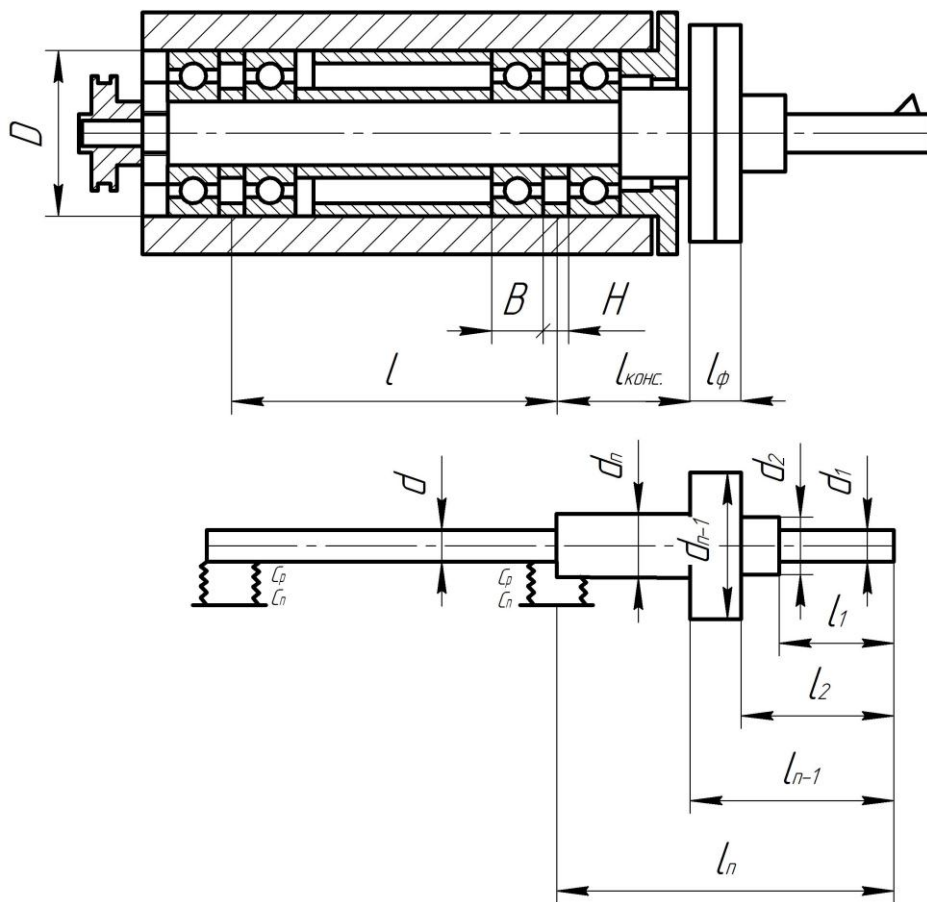
Рисунок 2 – Конструктивная и статическая расчетная схемы системы шпиндель-борштанга
