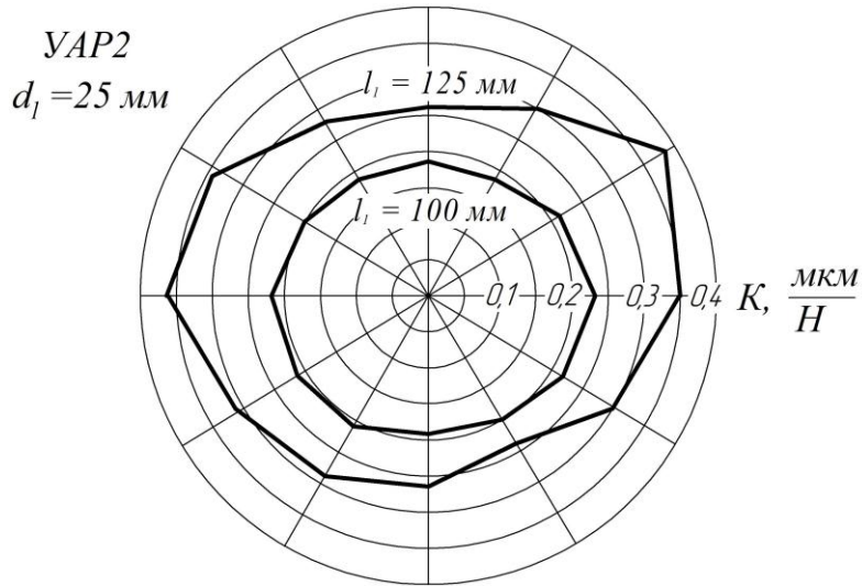
Рисунок 5 – Угловая эпюра радиальной податливости у резца
