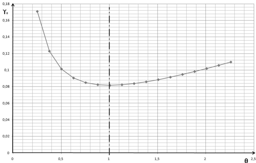
Рисунок 7 – Зависимость \gamma_0 от \theta
