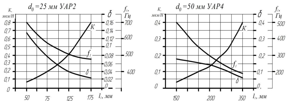
Рисунок 1 – Параметры системы шпиндель-борштанга f – первая собственная частота; \delta – логарифмический декремент колебаний
