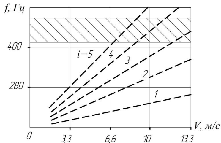
Рисунок 6 – Условия возникновения параметрических колебаний
