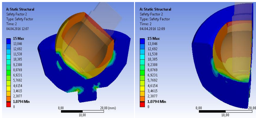
Рисунок 13 – Коефіцієнт запасу по першій теорії міцності для елементів, виготовлених з сафіру
