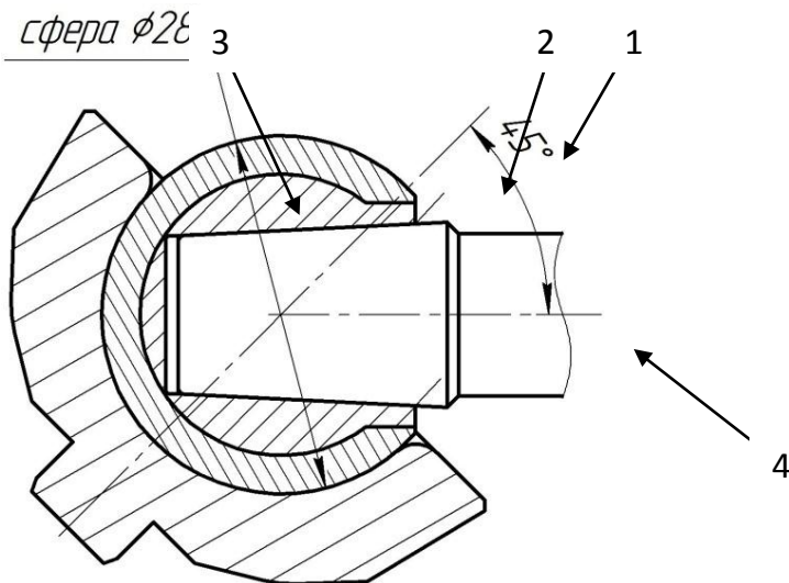
Рисунок 1 – Схема розташування елементів досліджуваної частини ендопротезу кульшового суглобу: двошарова головка (сферична оболонка з сапфіру – 1, серцевина з титану – 2), вкладиш ацетабулярної чаші – 3, посадковий конус ніжки – 4
