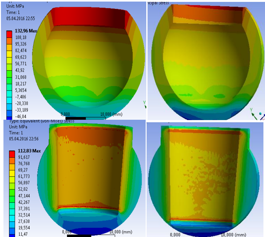
Рисунок 12 – Розподіл напружень при збільшенні довжини посадки конуса посадкового отвору
