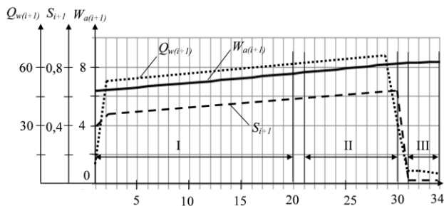
Рисунок 2 – Изменение параметров съема припуска: I, II, III – черновой; получистойвой и чистойвой этапы, соответственно
