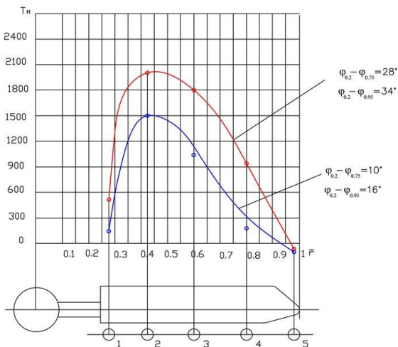
Рисунок 6 – Графік залежності тяги ВИГ от изменения крутки лопастей для максимального диаметра D_{\max} винта,
