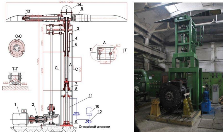
Рисунок 4 – Стенд динамических испытаний и фото стенда
