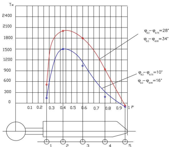
Рисунок 5 – График зависимости тяги ВИГ от изменения крютки лопастей
