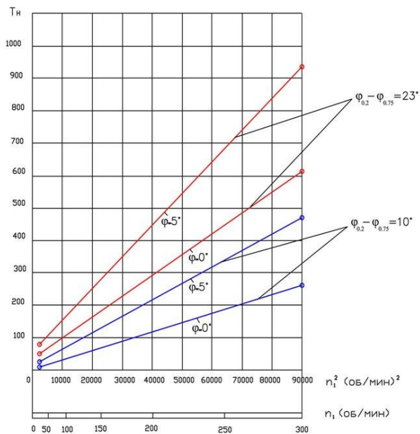
Рисунок 7 – Графік залежності тяги ВИГ от частоты вращения
