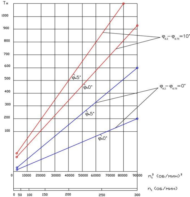
Рисунок 8 – График зависимости тяги ВИГ от частоты вращения винта, для максимального диаметра D_{\max}
