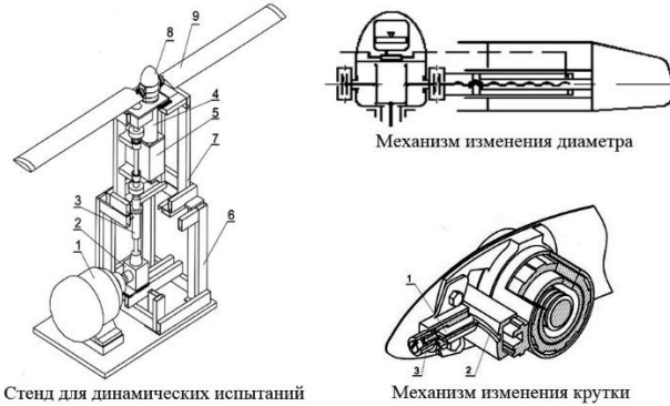
Рисунок 1 – Механизмы для управления параметров ВИГ-а и стенд для их испытания
