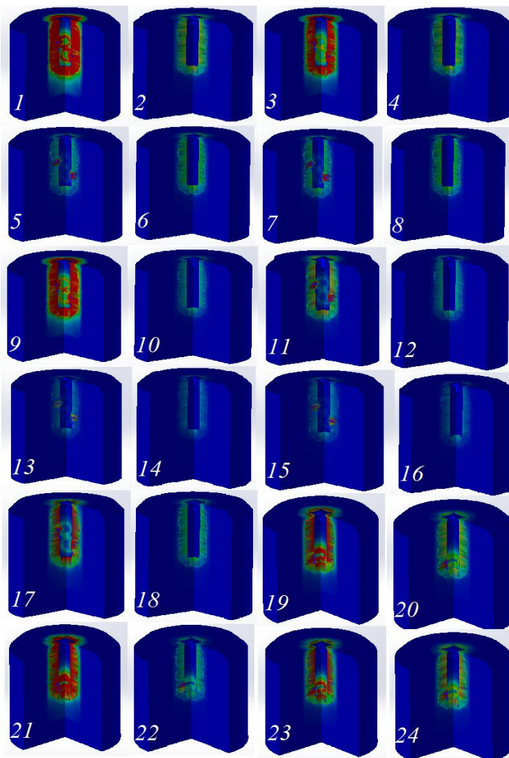
Рисунок. 1 – Визуалізація результатів моделювання НДС системи «металічне покриття – СПА – металлофаза»
