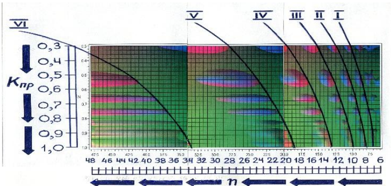
Рисунок 2 – Области параметрической неустойчивости упругой системы станка в виде эллипсов и границы зон устойчивой работы в виде кривых VI, V, IV, III, II, I. Расчеты произведены для t_a / t_\phi = 2 (для неимпрегнированного круга)
