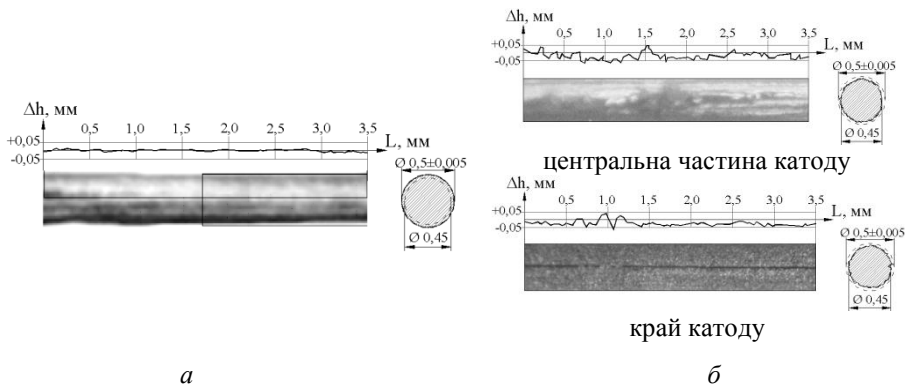
Рисунок 2 – Поверхня дротяного вольфрамового катода (діаметр D = 0,5 мм; довжина робочої частини L = 60 мм; струм розігріву I_f = 30 А; тиск p_0 = 0,5 \cdot 10^{-4} Па) до експлуатації (а) та після експлуатації (б) протягом 90 годин (78 циклів відкачування), профілограма та зображення отримані АСМ "NT-206V".
