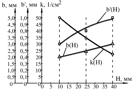
Рисунок 6 – Залежності ширини зони від термічного впливу b , центральної частини зони від термічного впливу b' і коефіцієнта зосередженості електронного потоку k_e від відстані до об'єкту дії ЕПГ H_{обр} .
