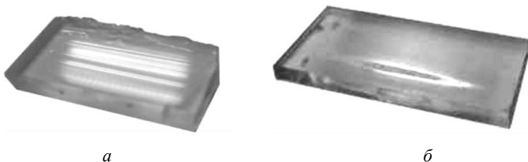
Рисунок 4 – Зовнішній вигляд поверхні кремнієвої пластини після дії електронного потоку: сканування по поверхні сформованим потоком (а); слід від нерухомого потоку ( T_0 = 600\text{ }^\circ\text{C} , U_{np} = 4\text{-}5\text{ кВ} , I_{nom} = 100\text{ мА} ) (б).
