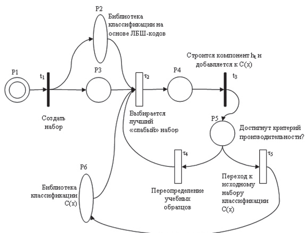
Рис. 1. Алгоритм распознавания
