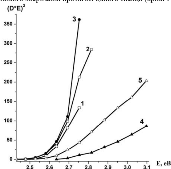
Рис. 2. Залежність від часу зберігання спектрів оптичного поглинання колоїдних розчинів нанокристалів CdS, отриманих за різної концентрації желатини, %: 2,5 (вихідні НК – крива 1; через 30, 45 дб – криві 2, 3), 1,7 (вихідні НК – крива 4; через 30 дб – крива 5).
