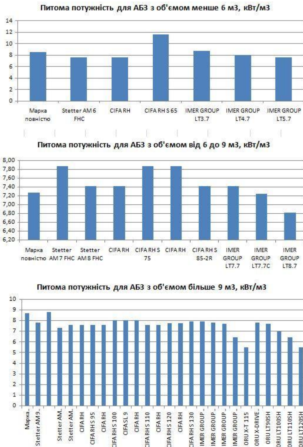
Рис. 18. Питома енергоємність.
