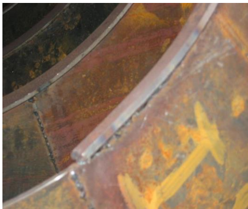
Рис. 5. Т-подібний захист (30x8 мм) на поверхні шнека барабанів фірми Stetter.
