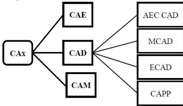
Рис 2. Класифікація CAx-систем.
