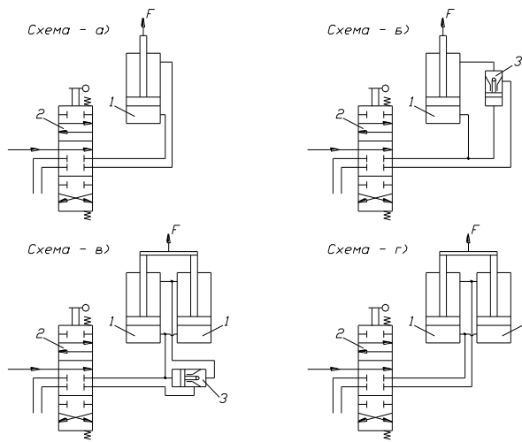
Рис. 1. Гідравлічні схеми під'єднання гідроциліндрів в функціональних дільницях: 1-гідроциліндр; 2-гідророзподільник, 3-гідрозамок або клапан керування зворотній.
